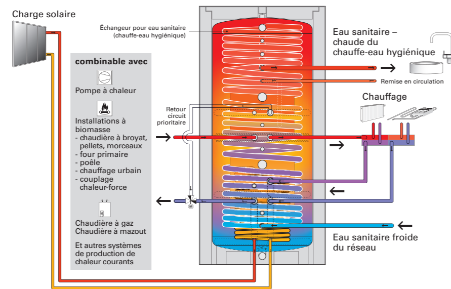
L'accumulateur Forstner HS ne produit pas de la chaleur, mais il l'accumule, la stratifie, la régule, la gère et la distribue.
